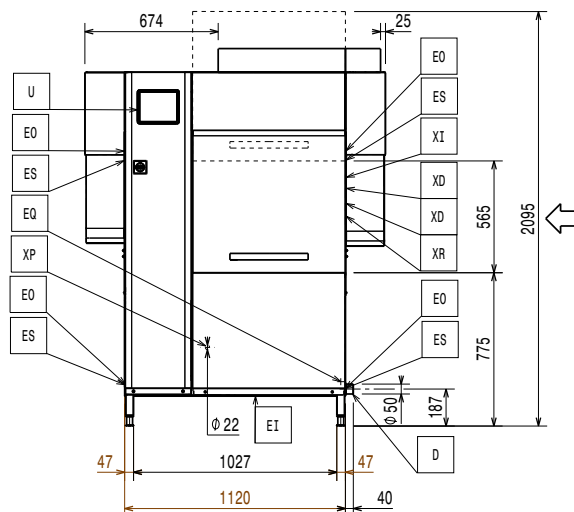
Boční
